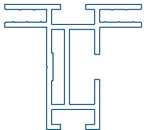
FitFRAME duo50
